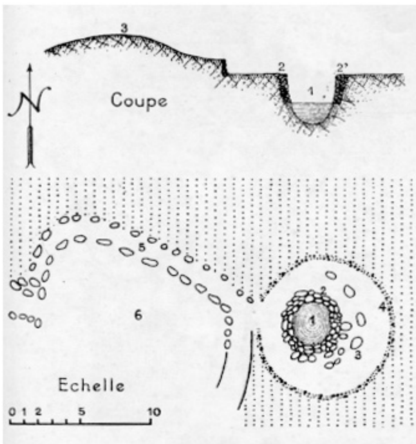
Planche CLXXVIII. — Puits Đống. Village de Liêm - Công - Tây — Coupe : 1, puits. 2, 2', parois. 3, autel champêtre moderne.
