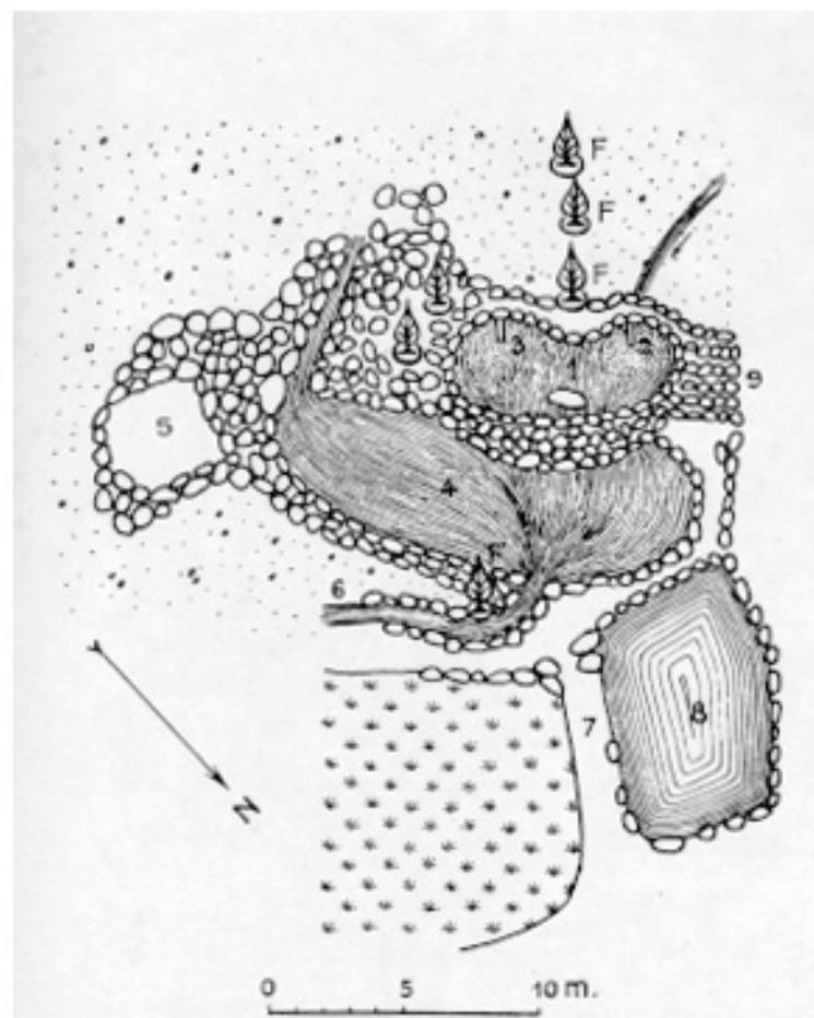
Planche XCIV. — Bassins Sôï ( village de Hào -Son ) — Plan : 1, bassin de réception et d'alimentation. 2 et 3, becs de cuve. 4, grand bassin. 5, petit terrasse. 6, défluent. 7, diguette. 8, bassin stagnant. 9, escalier. F = Ficus.
