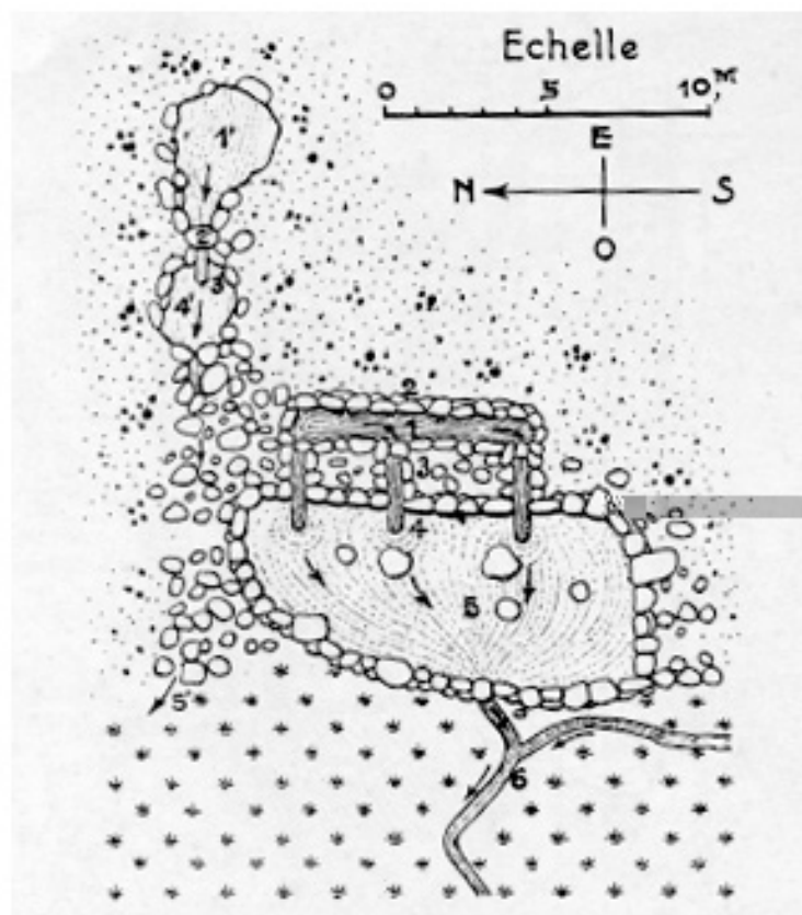
Planche LXXV. — Plan : A droite, bassin Trang ; en haut, à gauche, bassin Bång ( village d'An -Nha ) — Bassin Trang : 1, bassin supérieur. 2, mur. 3, terrasse sèche. 4, bec de cuve. 5, bassin d'alimentation. 6, déversoir. ( Voir Pl. IX.) Bassin Bång : 1', bassin supérieur. 2', pont. 3' bec de cuve. 4' bassin d'alimentation. 5', sortie de l'eau.
